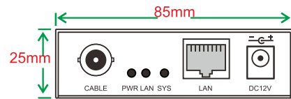
前视图
