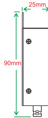
侧视图
